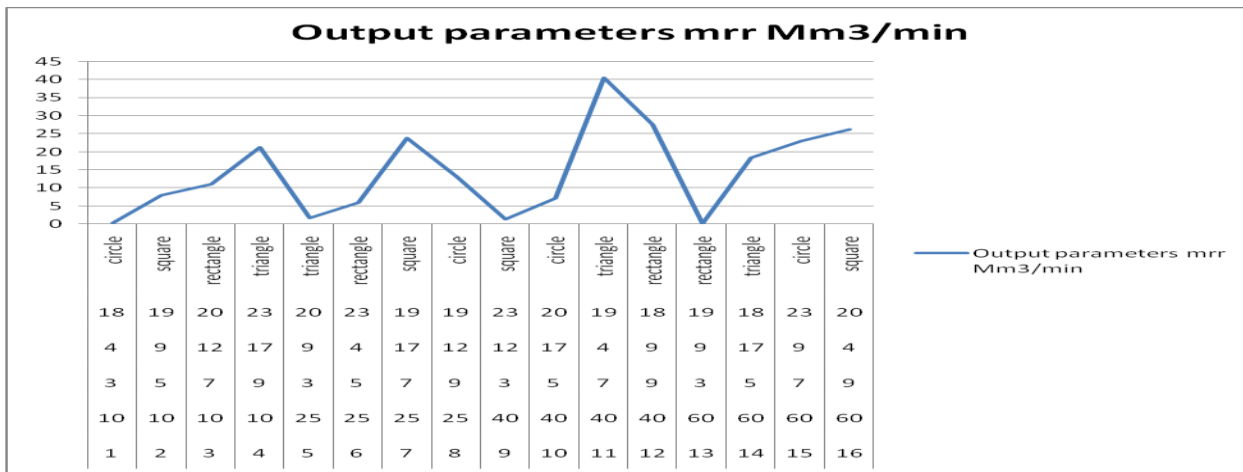
FIG.2 OUTPUT PARAMETERS OF TWR
