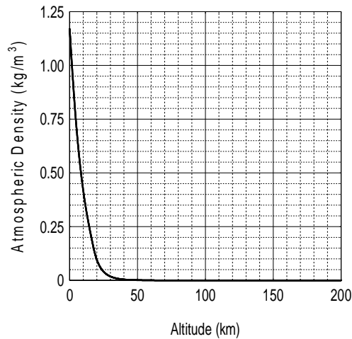
Fig.7. Altitude Vs. Density
