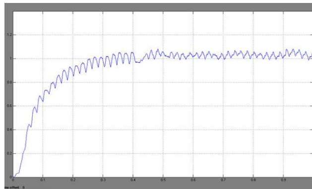
Fig. 10. DC-link voltage of AVSI
