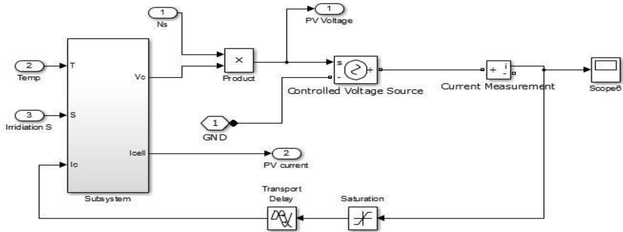
Fig. 5 Solar module Simulink design
