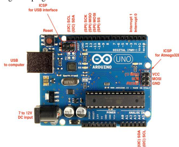
Fig. 2 Arduino ATmega328
