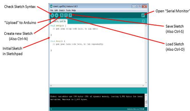
Fig. 3 Arduino IDE[12]
