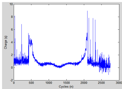
Fig.9 (d) Skewness plot (n-q) of corona discharge
