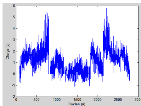
Fig.12 (d) Skewness plot (n-q) of data3
