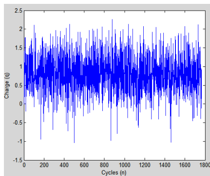
Fig.8 (d) Skewness plot (n-q) of surface discharge
