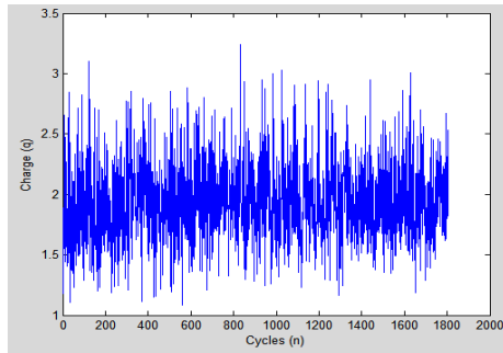
Fig.11 (d) Skewness plot (n-q) of data2
