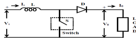
Fig 6 : Boost Converter
