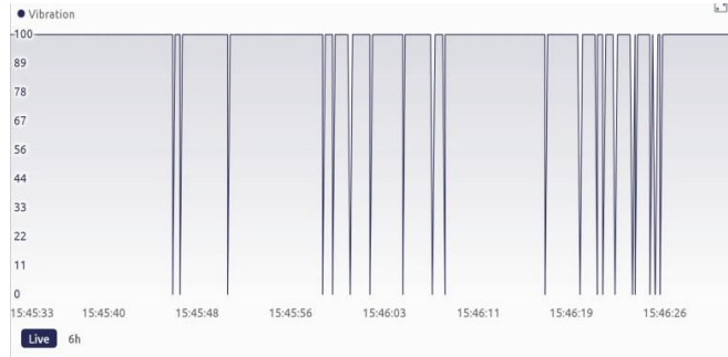
FIG.NO.4 UN DAMAGE CUBE VAIBRATION GRAPH
