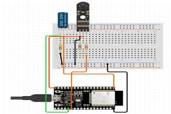
FIG.NO. 1 CIRCUIT DIAGRAM
