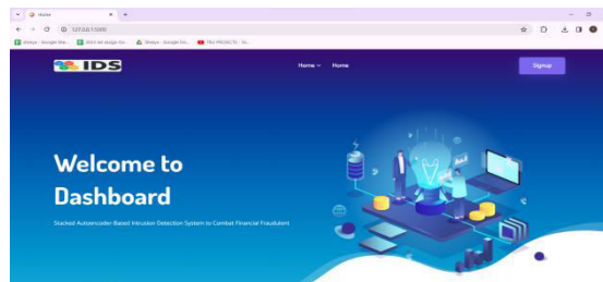
Fig 13 Web page
