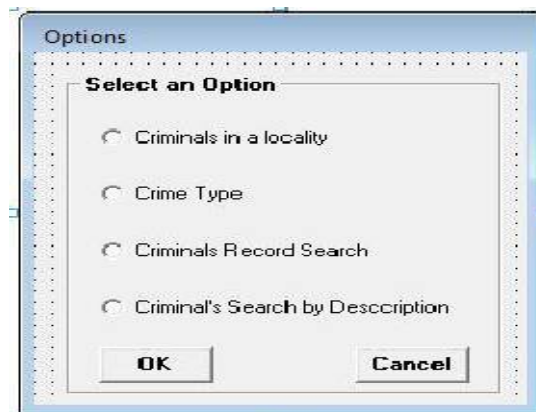
Fig 3. Options Dialog
