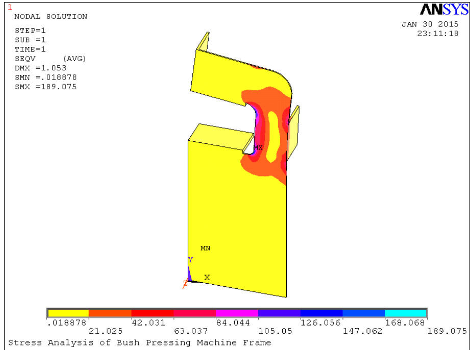
Fig. 12 Von Mises Stresses
