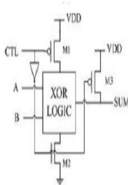
Fig.4.Modified XOR Gate
