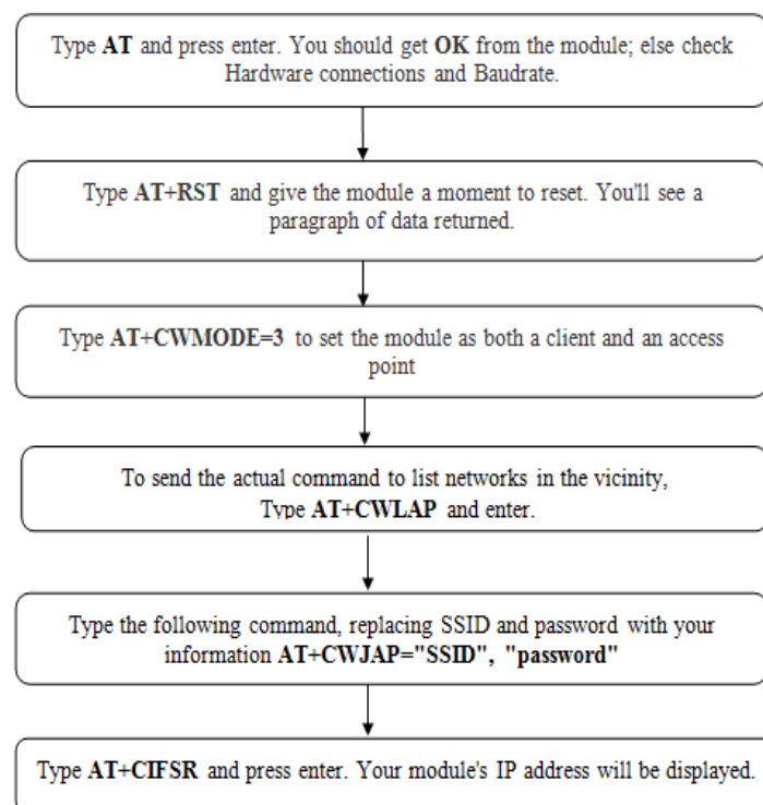
Fig.8. Configuring the ESP8266 Module
