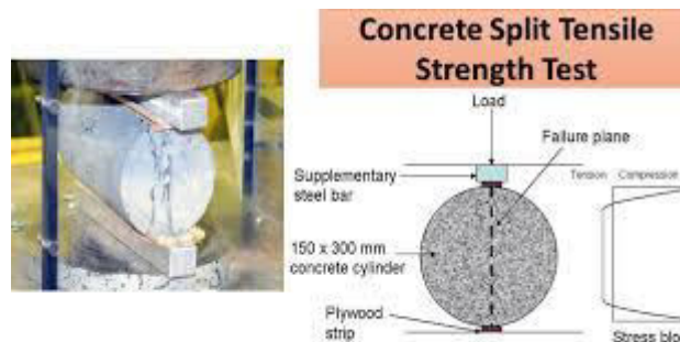
Fig.3 Split Tensile Test
