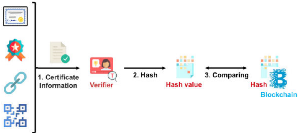
Fig 3: Step 3 (Verify)
