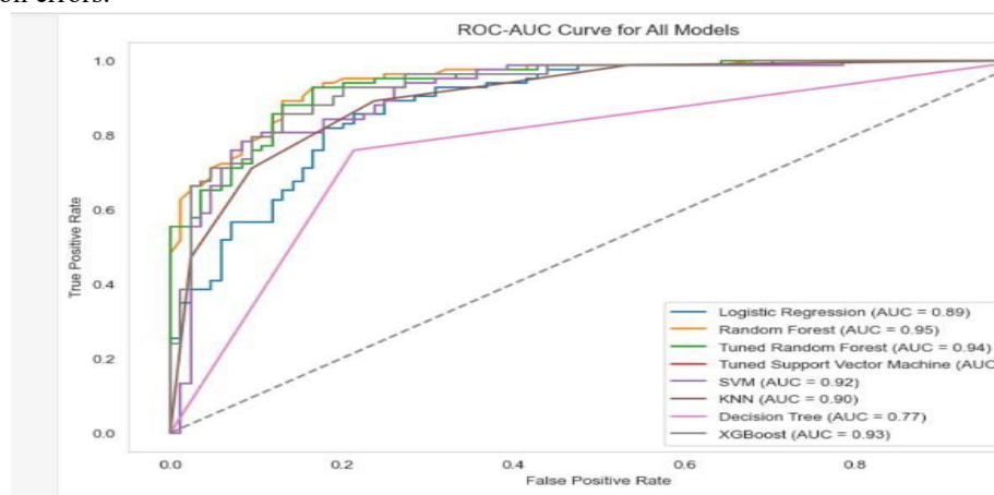
Fig. 4. AUC – ROC curve
